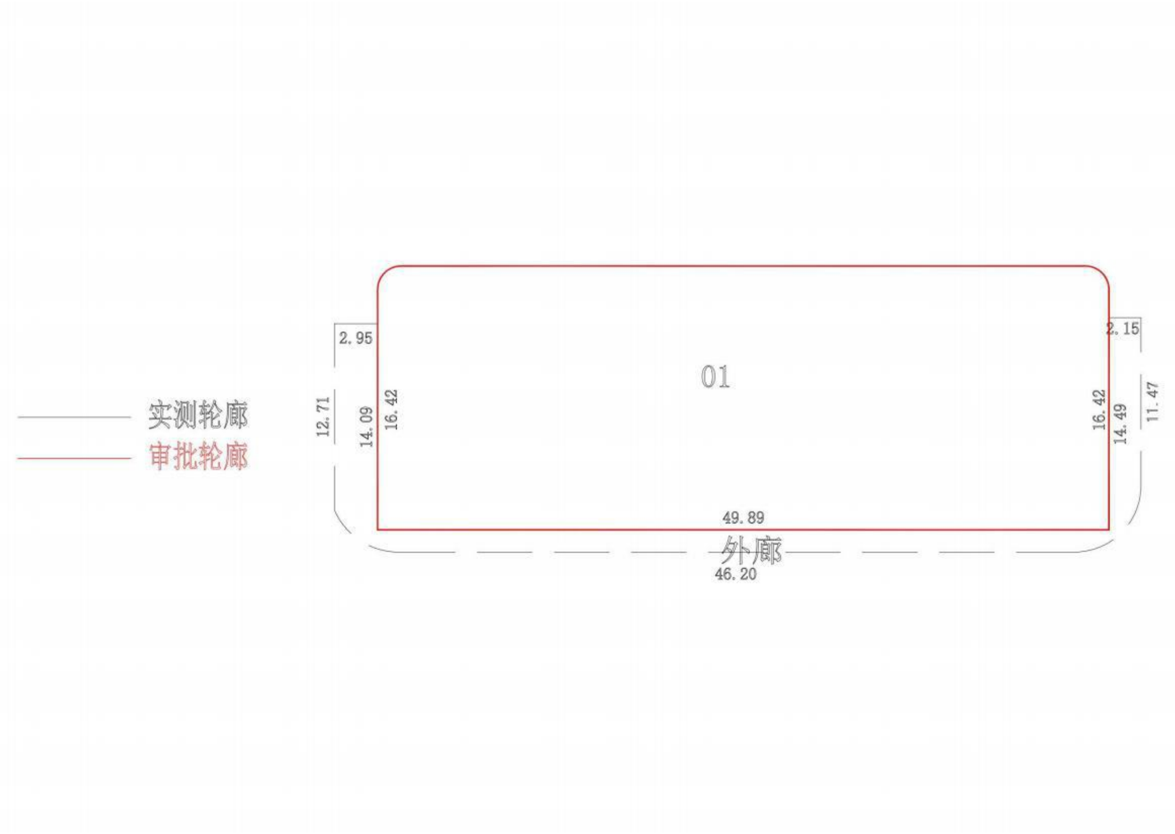
实测分层图对比二层
