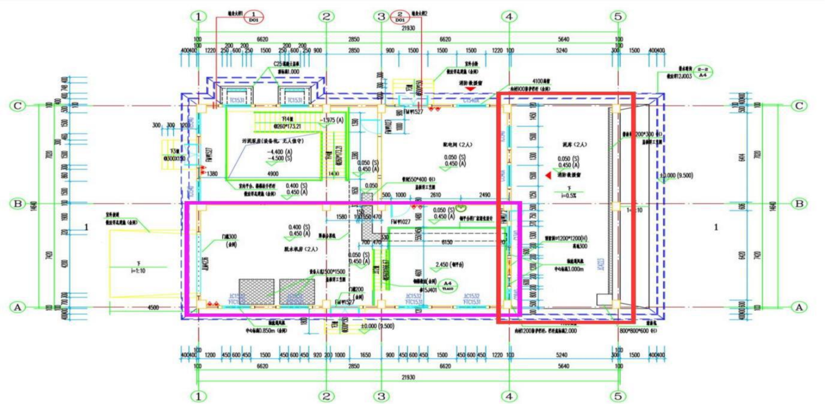
设计施工图
